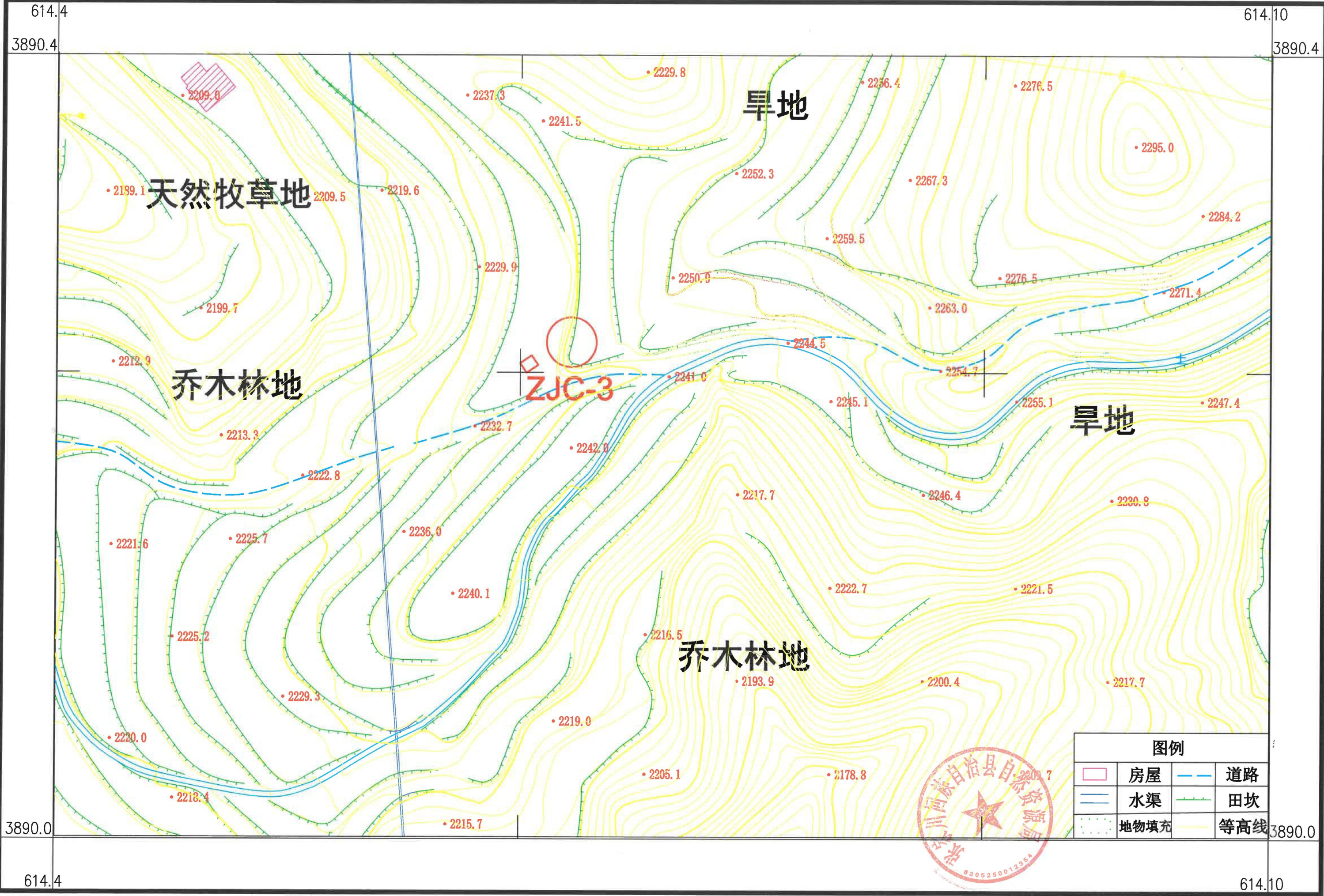
张家川县新华一期50MW风电项目范围图(ZJC-3)
