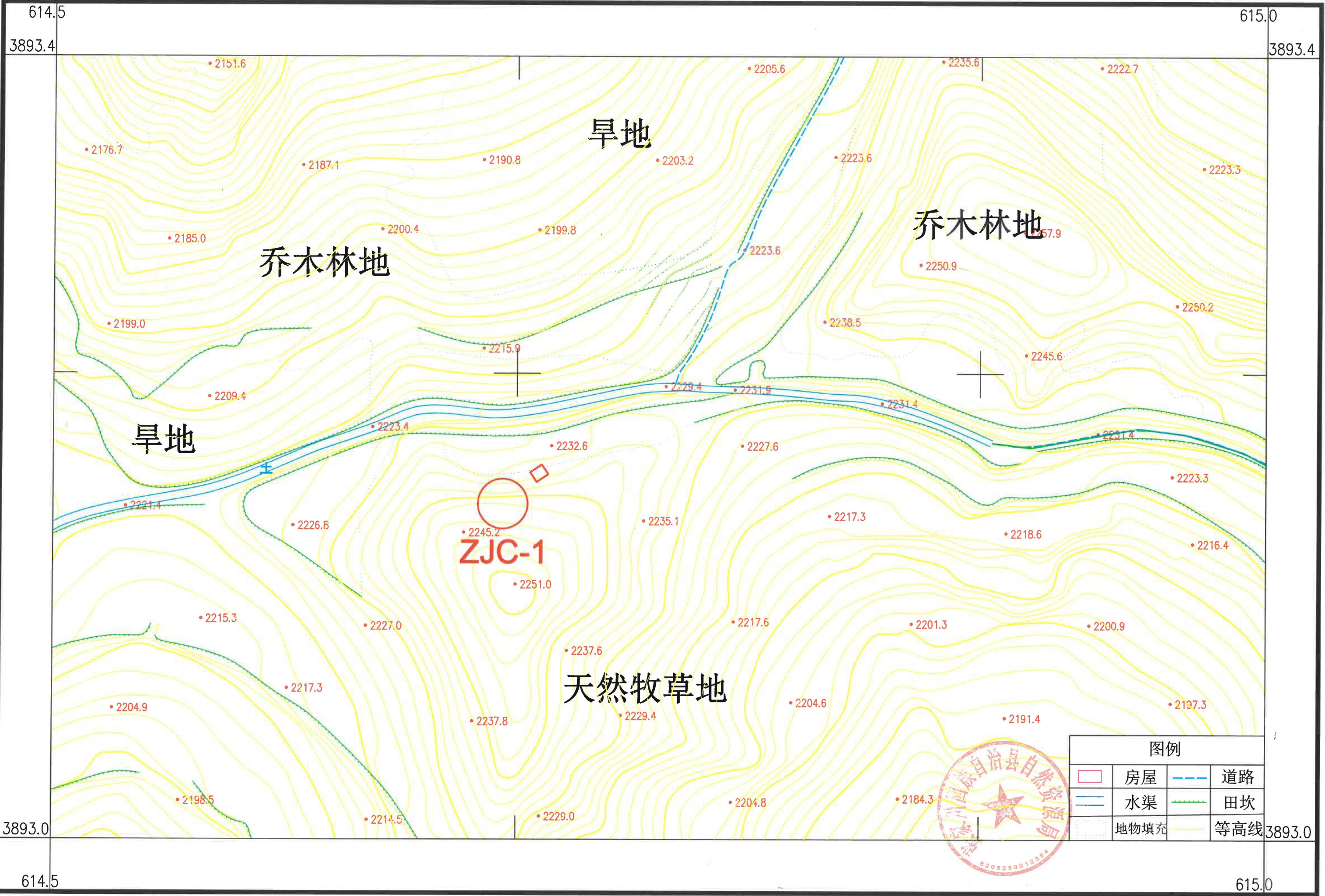
张家川县新华一期50MW风电项目范围图(ZJC-1)
