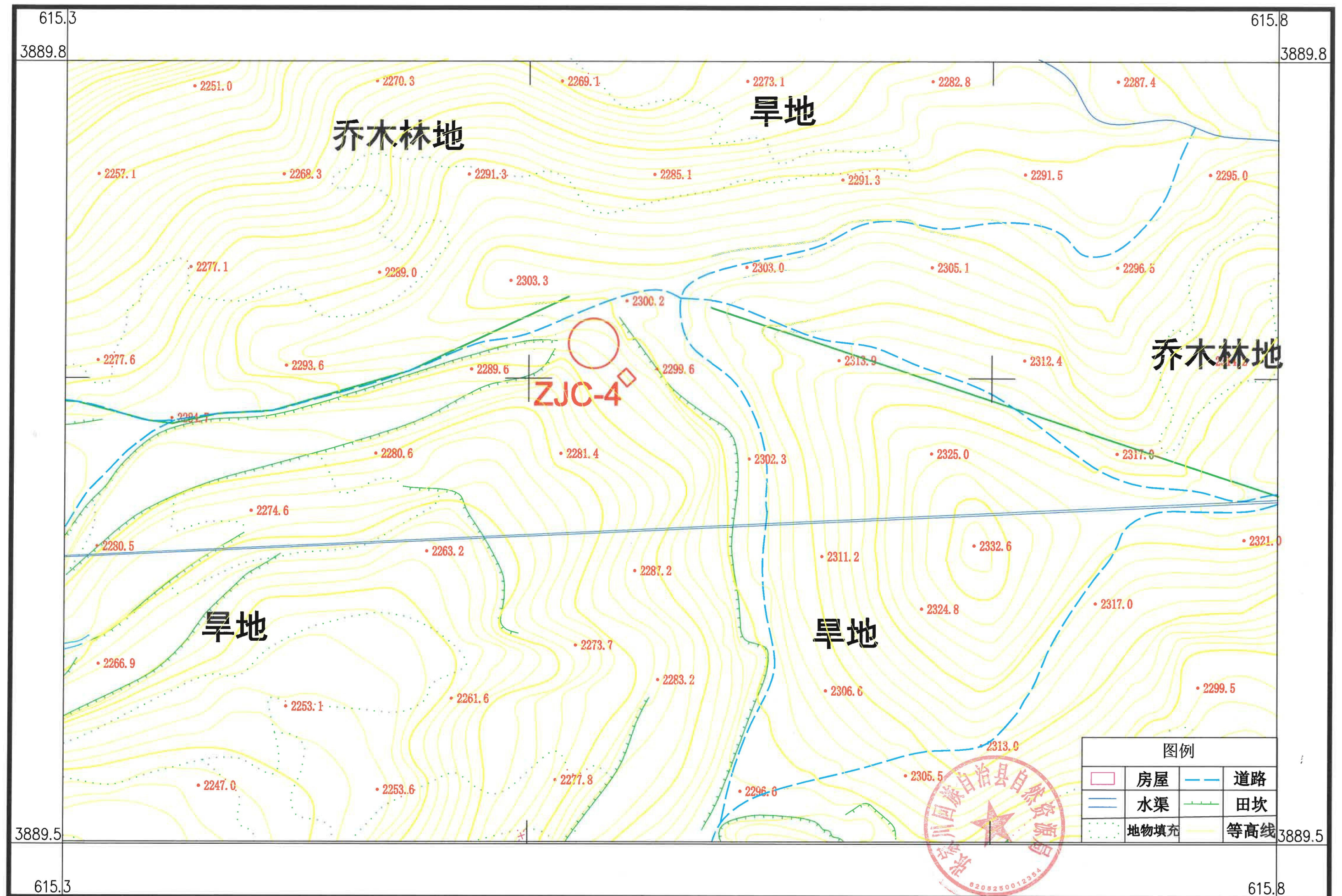
张家川县新华一期50MW风电项目范围图(ZJC-4)
