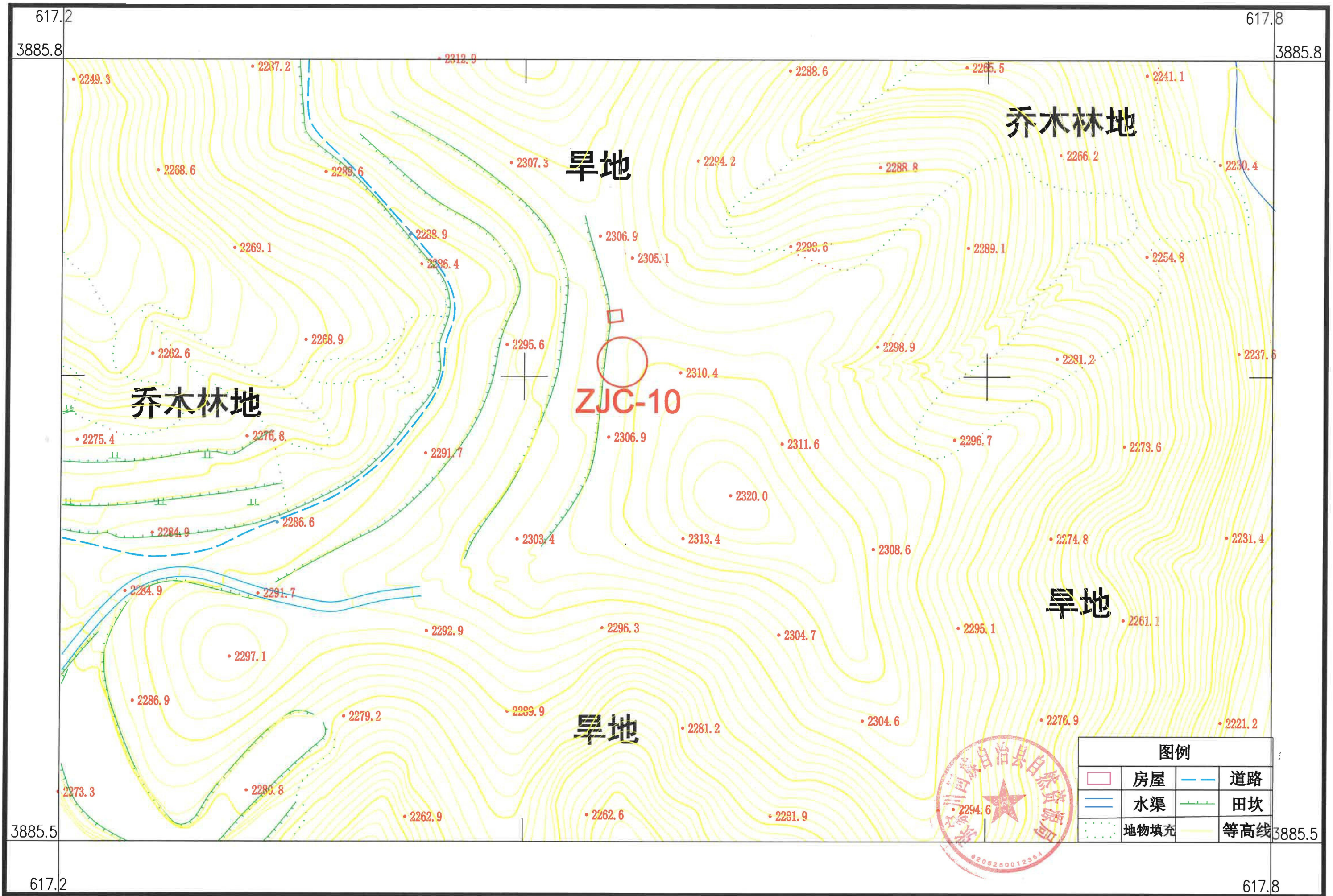
张家川县新华一期50MW风电项目范围图(ZJC-10)
