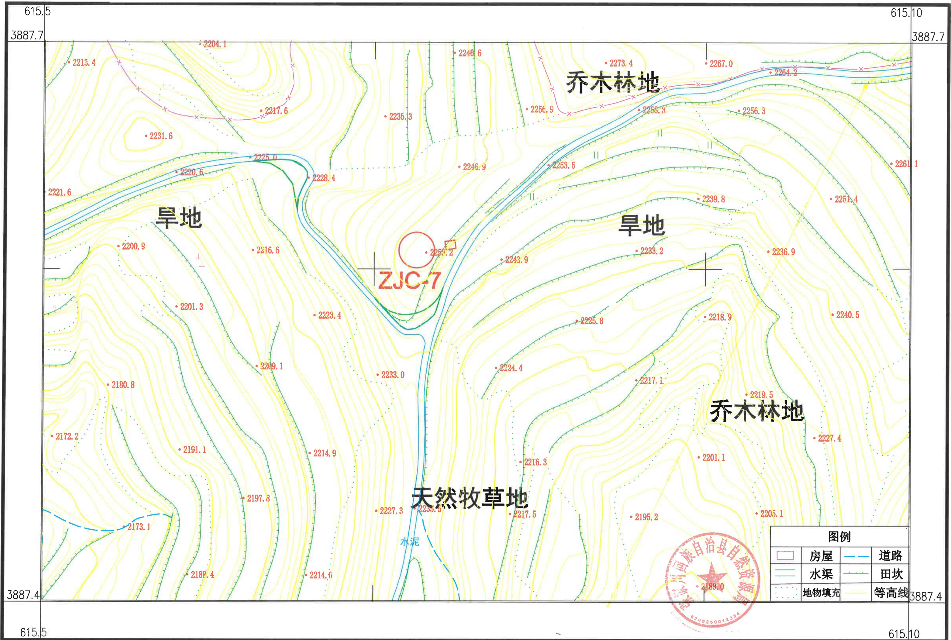
张家川县新华一期50MW风电项目范围图(ZJC-7)
