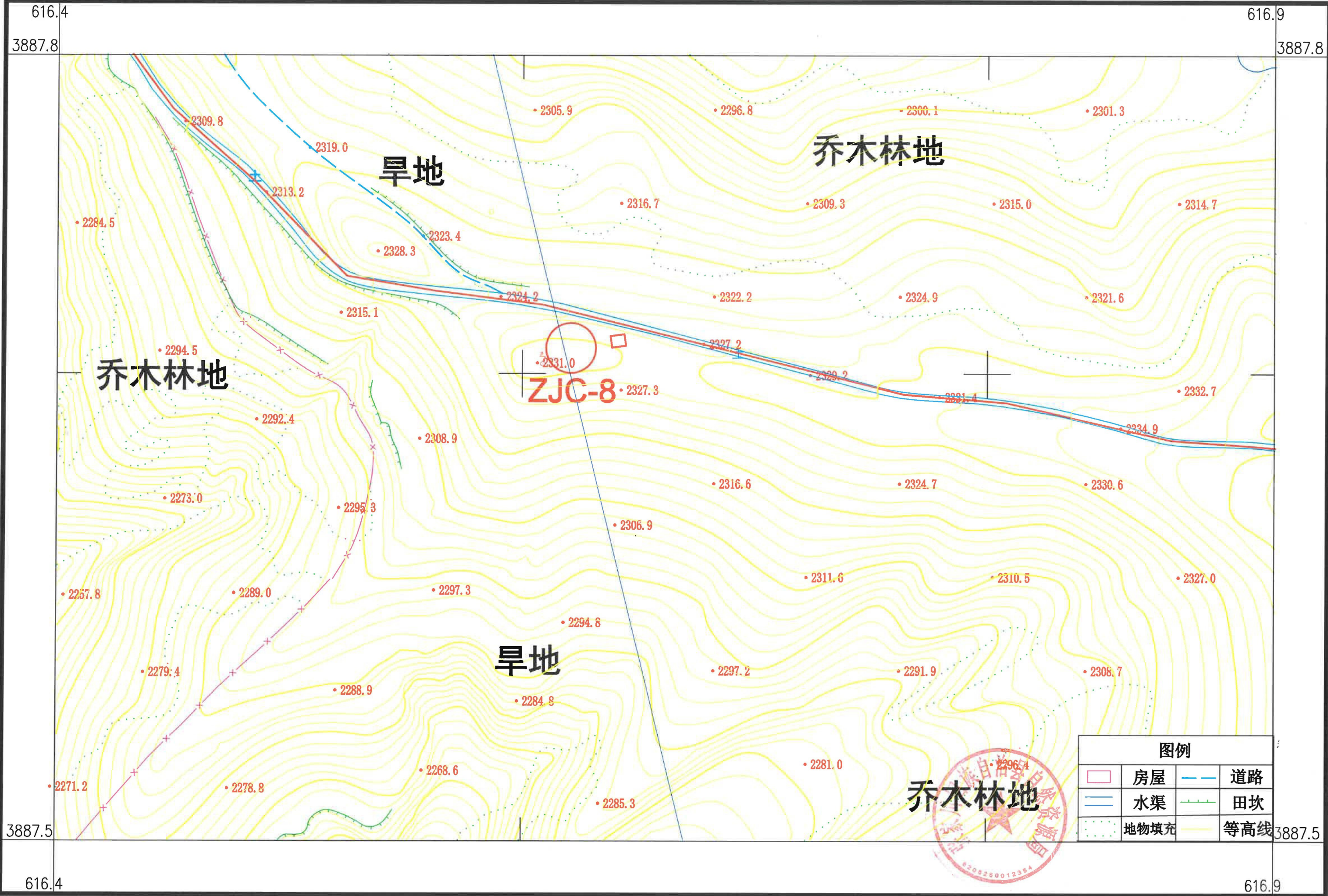
张家川县新华一期50MW风电项目范围图(ZJC-8)
