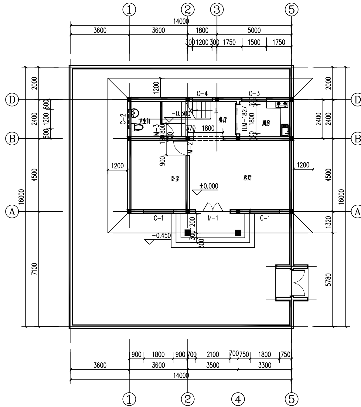
院落平面图 1:100
